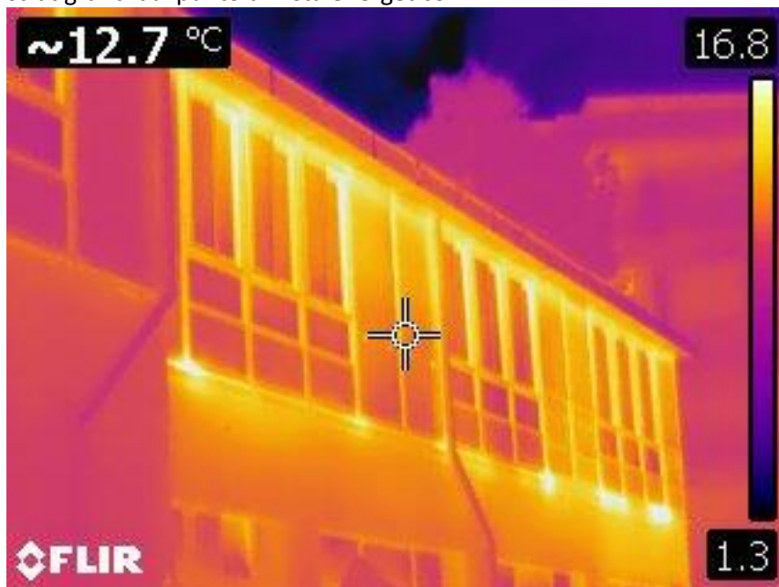
Figura 2.2 – Immagine termografica facciata - solaio interpiano
