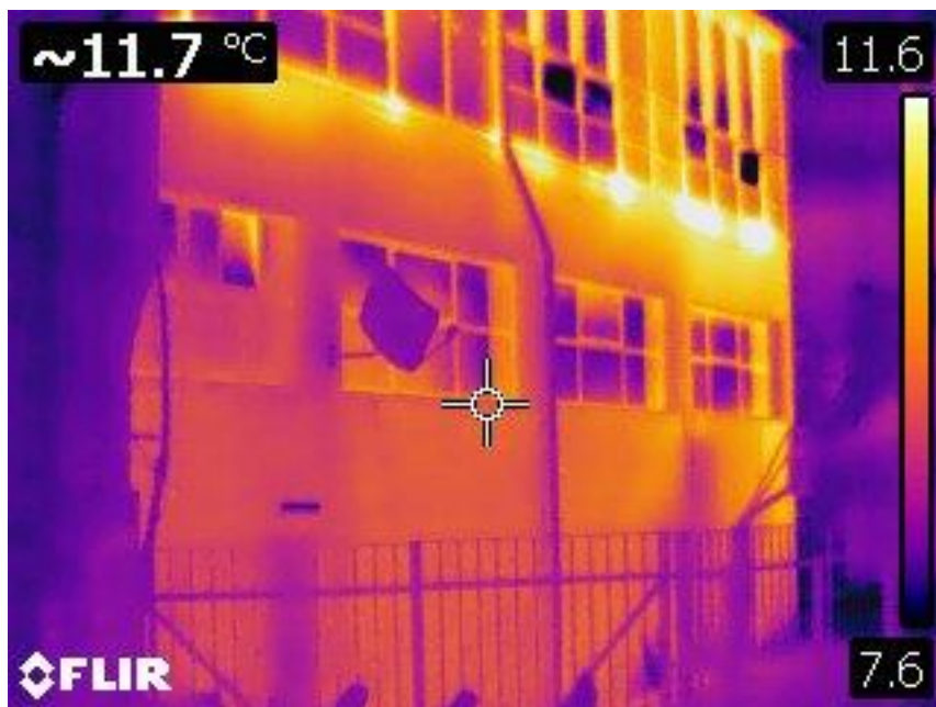
Figura 2.3 – Immagine termografica facciata
